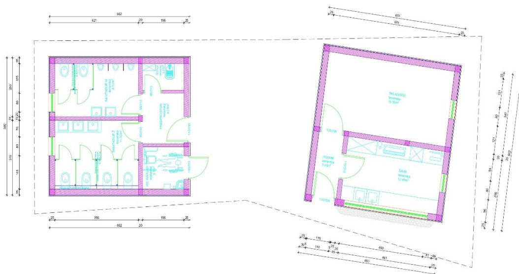
SLIKA 2: TLOORIS NOVE ZGRADBE, LETNI KINO
