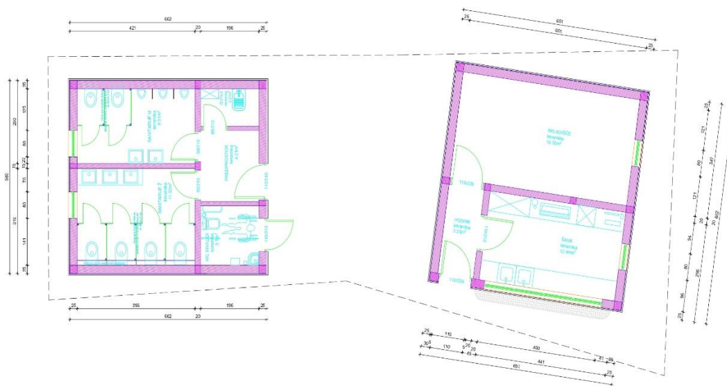
Slika 2: Tloris nove zgradbe, Letni kino
